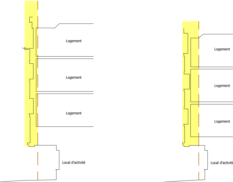
Coupe A-A'
